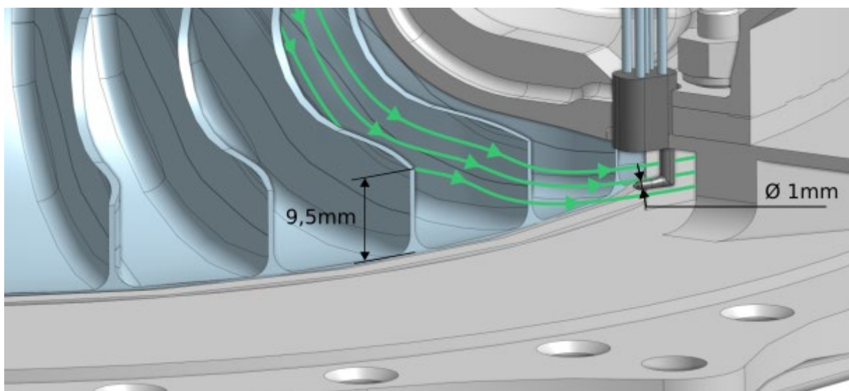
Abbildung 1 – CAD-Anordnung einer Strömungsmesssonde In einem Radialkompressor. Lauftrad (blau), Diffusor (grau, aufgeschnitten)
